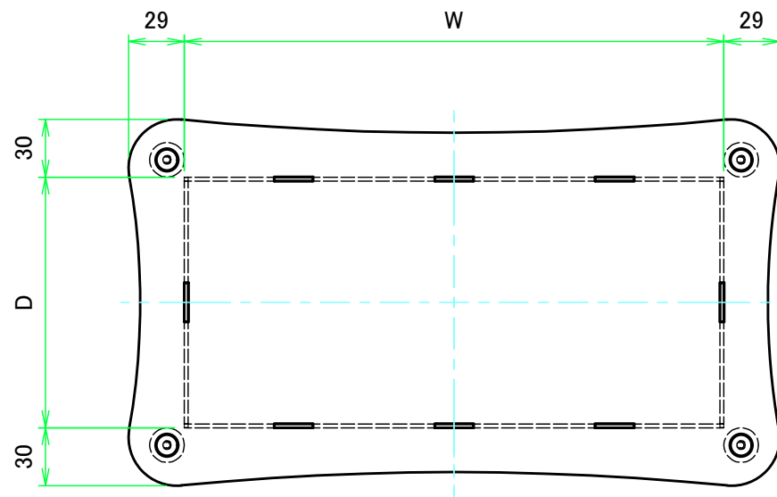
上カバー / Top cover
