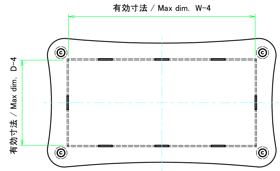
下カバー / Bottom cover
